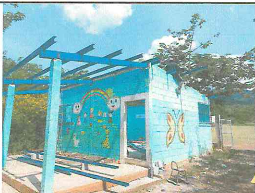
FOTO 3: INSTALACIÓN DE ESTRUCTURA DE METAL.
